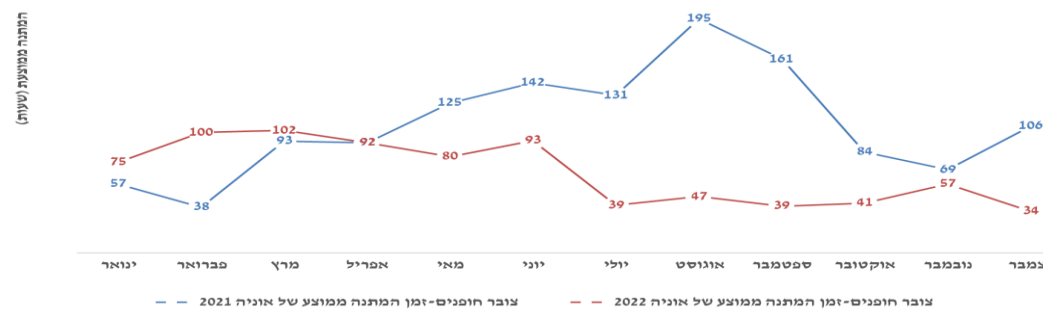
זמן המתנה ממוצע לאוניות מתקנים - נמל מספנות ישראל
