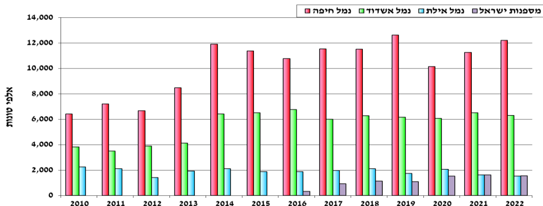
תנועת מתקנים אוטומטיים בנמלי המסחר 2010-2022
