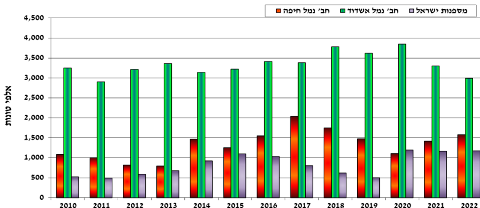
תנועת צובר חופנים בנמלי המסחר 2010-2022
